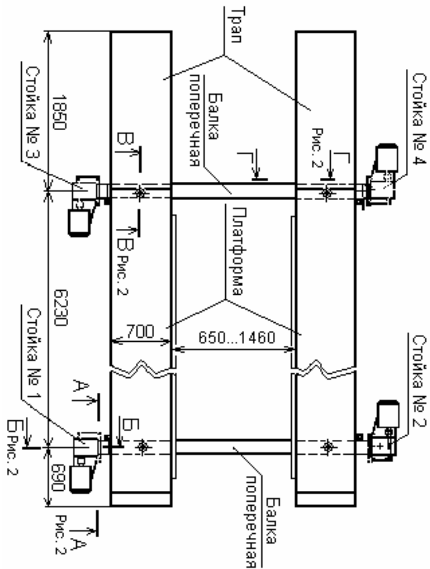
Рис. 1. Подъемник ПЛ15
